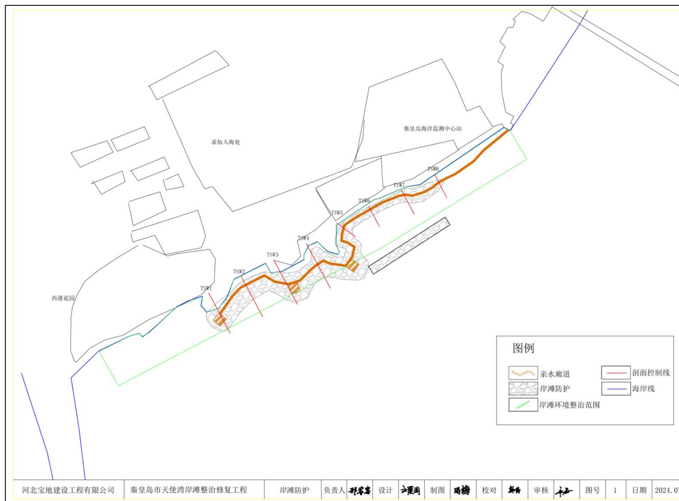
图 2.2.1-1 本项目总平面布置图 (**坐标, **高程)
